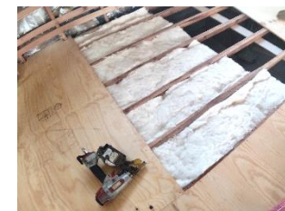
断熱材の設置事例
