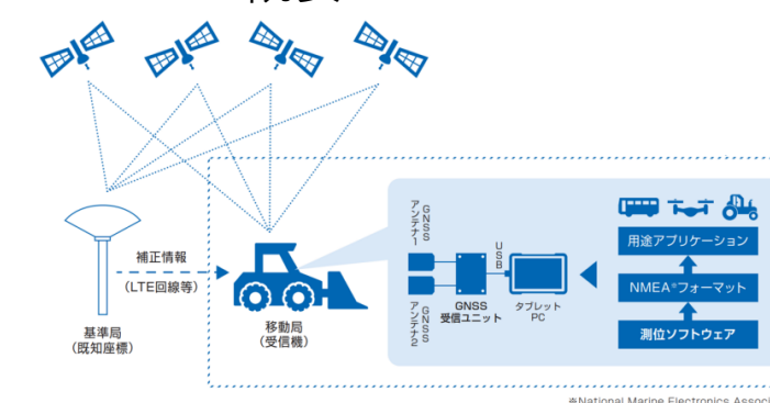
土木・建機
