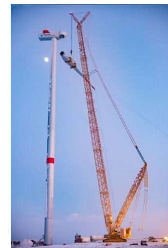
陸上で風車のブレード据付を行うCC
