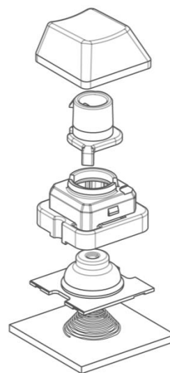
静電容量無接点方式キー断面図
